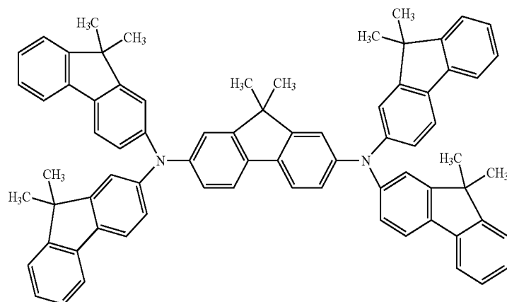
TFLFL
