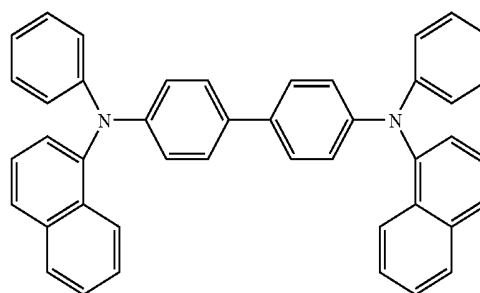
\alpha -NPD
